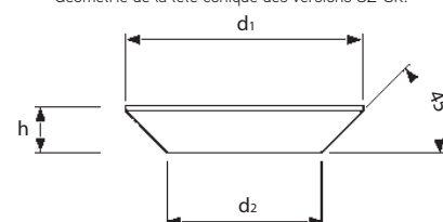
Géométrie de la tête conique des versions SZ-SK.
